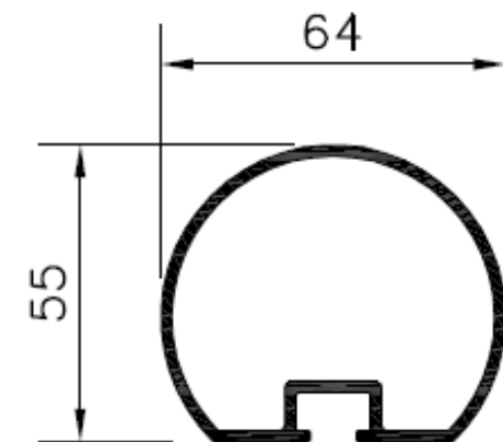
Handregelprofiel 64-55
