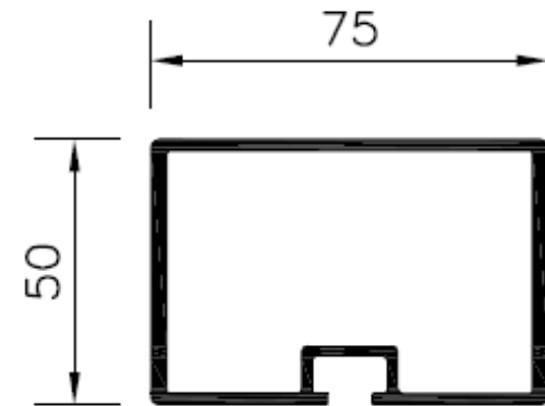
Handregelprofiel 75-50
