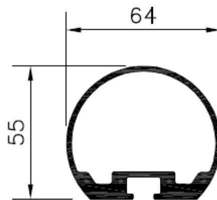
Handregelprofiel 64-55Z
