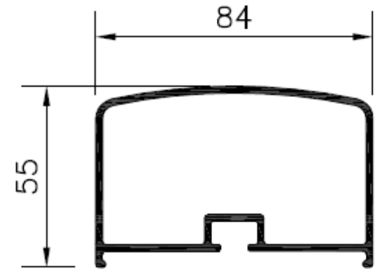
Handregelprofiel 84-55
