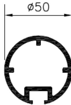
Handregelprofiel Ø50
