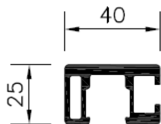
Glashekprofiel 60-48T
